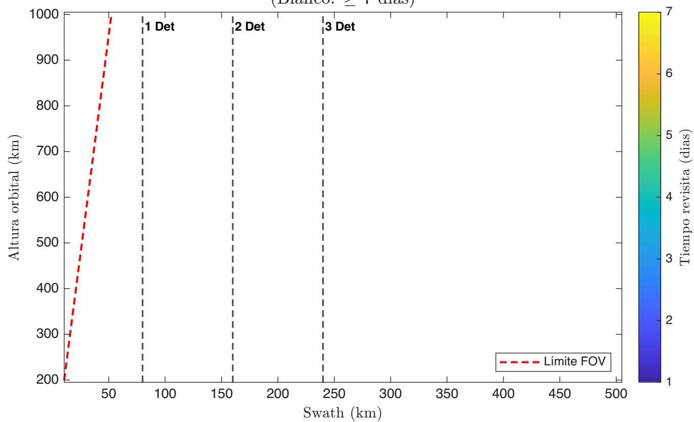
Tiempo Revisita - 2 Satellite(s); 1 Telescopio(s): Korsch; Detector 3 (Blanco: \geq 7 dias)
